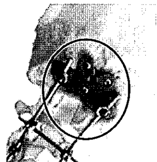
蝴蝶型枕骨板
