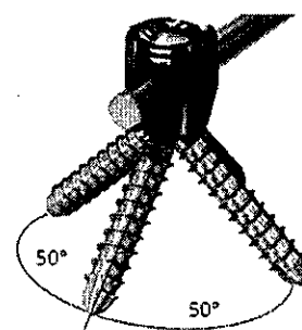
本案之頸椎固定螺釘：多向式
