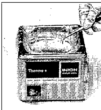
骨板加溫塑形以符合骨骼斷面
